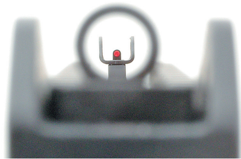
Фотоснимок не совсем точно передаёт картину, видимую через прицел «Каратая». При прицеливании кольцо диоптра размывается ещё больше, не перекрывая поле зрения
