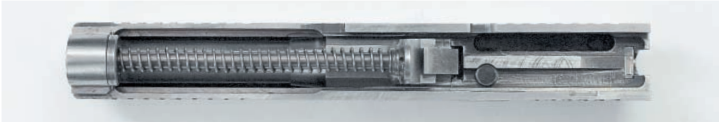
Затвор ПЕ-9 со стволом и возвратным механизмом. Вид снизу
