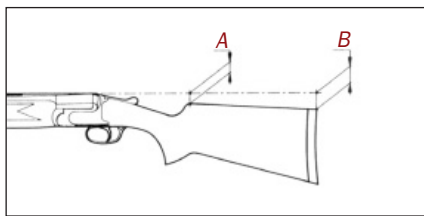
Погиб ружья характеризуется высотой гребня приклада в передней (А) и задней (В) точках
