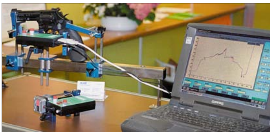
Небольшой стенд для измерения характеристик спуска подключается к портативному компьютеру, давая возможность сравнить полученные данные с эталонной кривой
